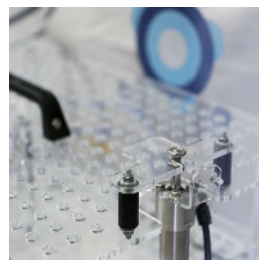
Panier sur verin pneumatique pour test d'immersion non destructif
